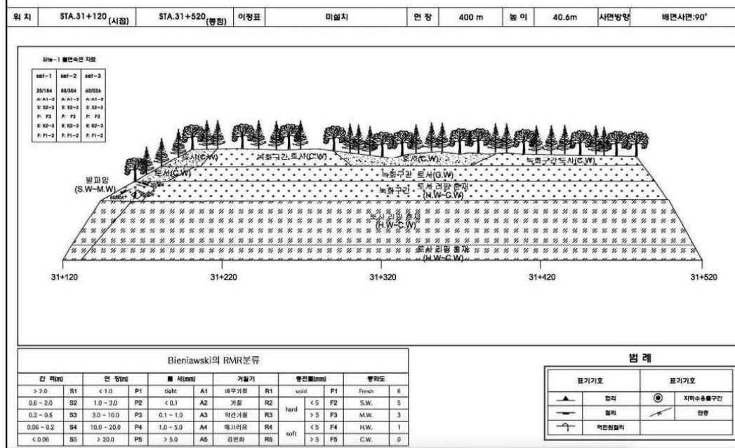
깎기비탈면 현황도(내포리구간(좌안) : 내포육교 전 STA.31+120~31+520)
