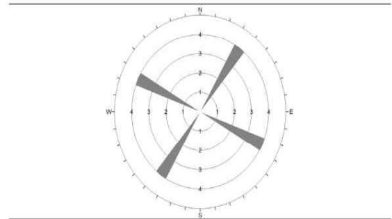
〈그림 16〉 Site-1 절리분포 현황
