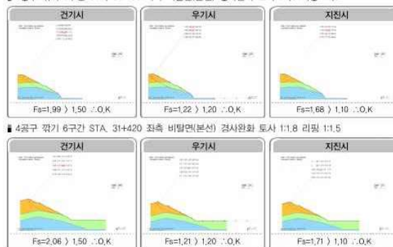
■ 4공구 깎기 6구간 STA. 31+180 좌측 비탈면(본선) 경사완화 토사 1:1.8 리핑 1:1.5
